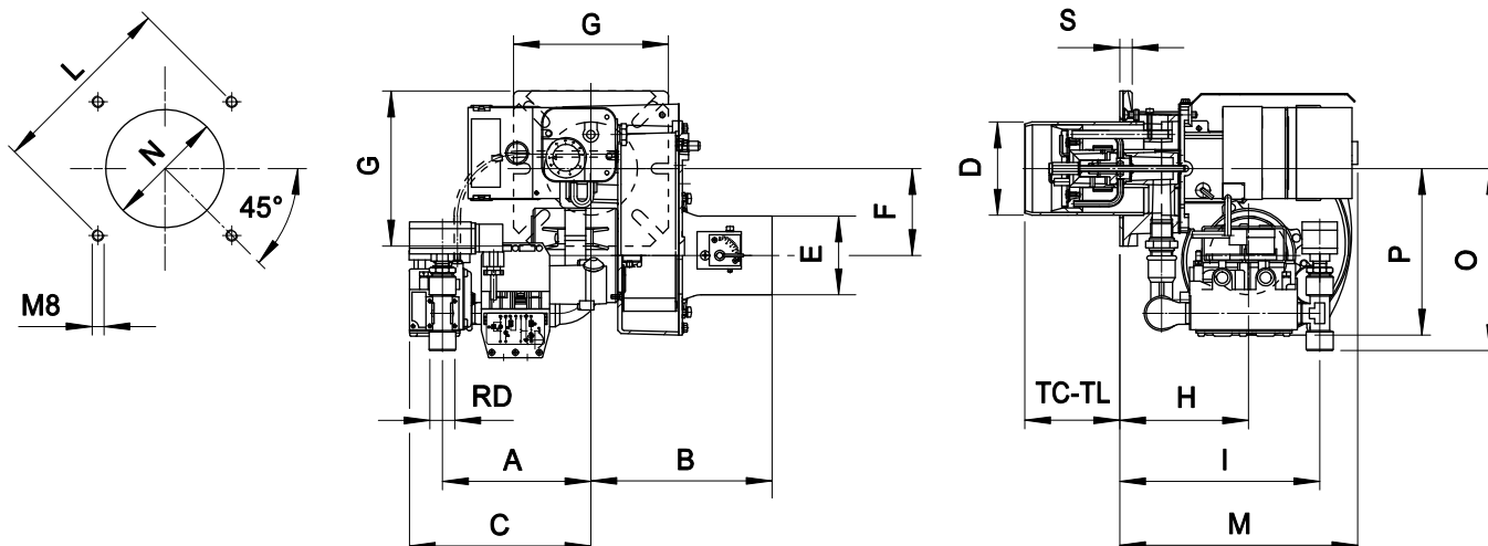
РАЗМЕРЫ [мм]
